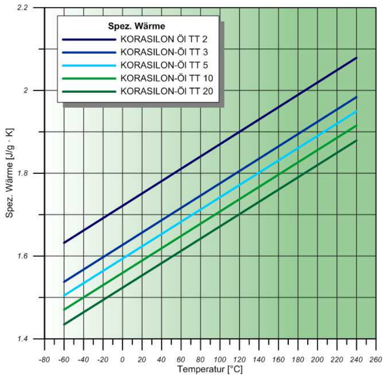
Temperaturabhängigkeit der spezifischen Wärme
